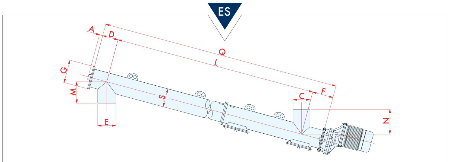
Riduttore: - Costruzione per servizio pesante - Ingranaggi sovradimensionati
